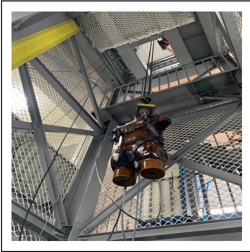
全身背負式安全帶性能試驗
